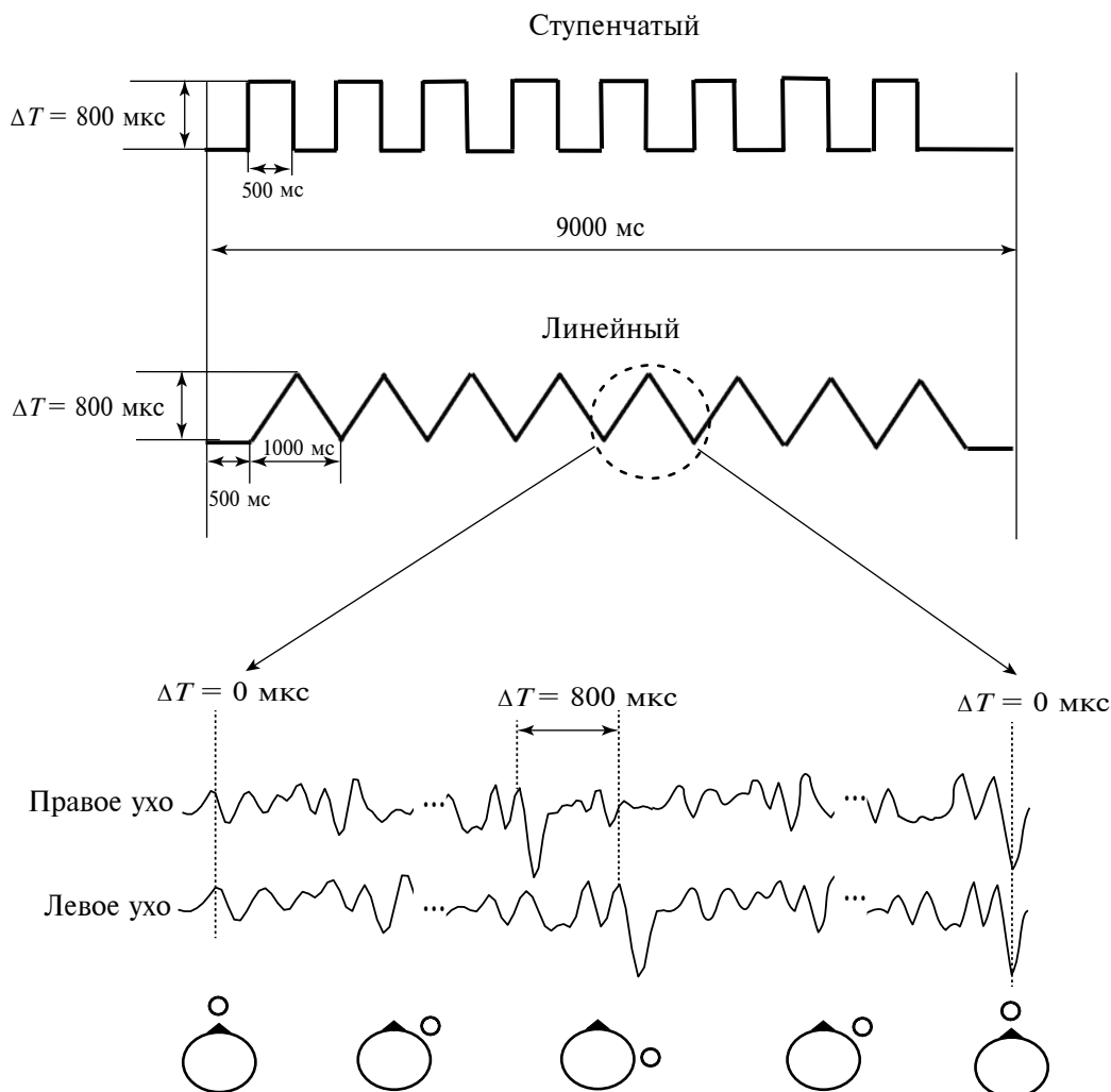
Рис. 1. Изменения величины межушной задержки в бинауральных звуковых стимулах, моделирующих плавное и ступенчатое циклическое движение. Вверху: временная структура стимулов в пределах одной пробы. По горизонтали — время (мс), по вертикали — величина межушной задержки ( \Delta T , мкс). Разные начальные значения \Delta T определяют разные положения траекторий циклического движения в субъективном слуховом пространстве. Внизу: схема дихотической стимуляции в одном цикле линейного паттерна (от 0 мкс до 800 мкс и обратно к 0 мкс). На схемах головы условно изображено последовательное изменение положения звукового образа в соответствии с изменениями \Delta T .
